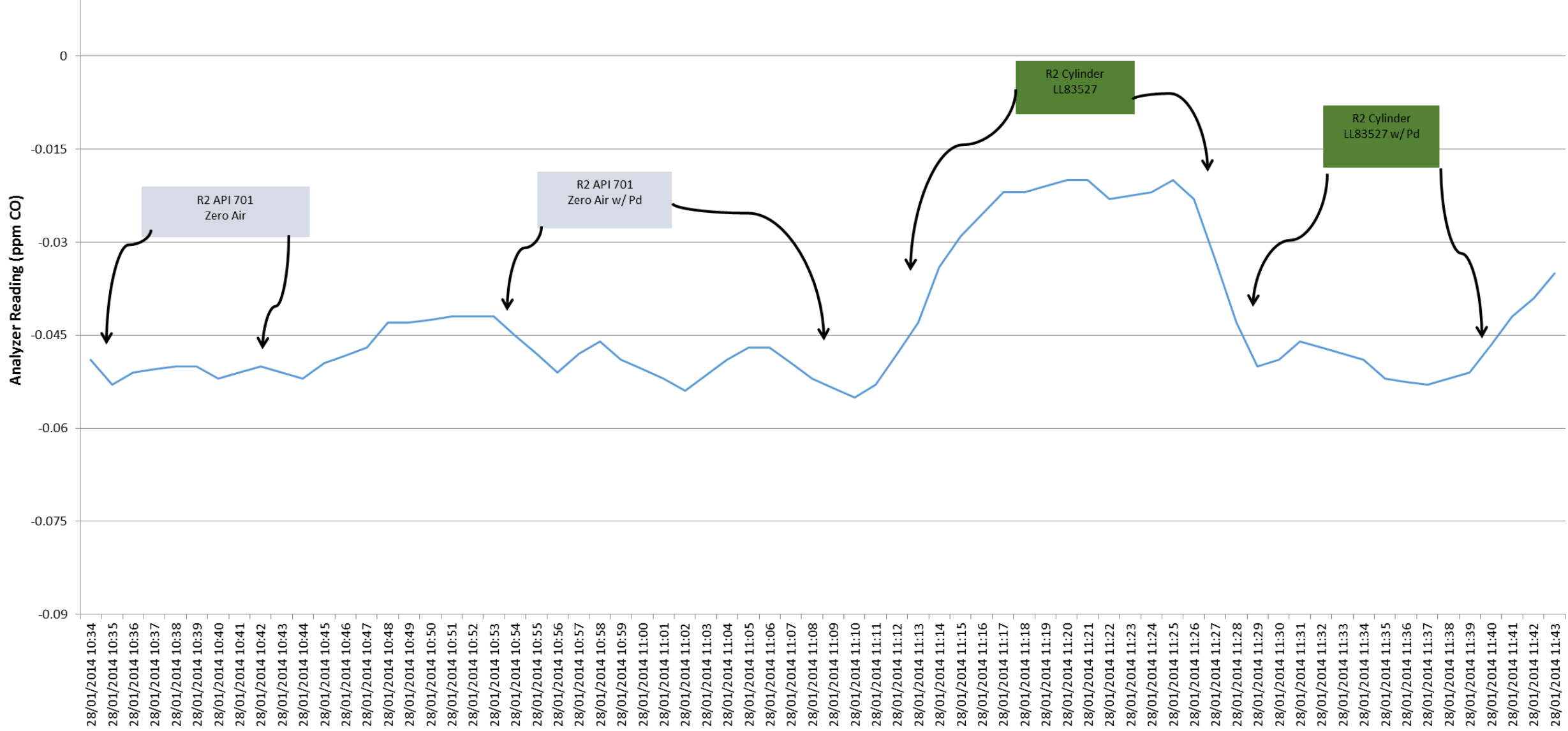
TTP CO Baseline - R2 API 701 vs. R2 API 701 w/ Pd Scrubber vs. R2 TTP Zero Gas Cylinder Standard
